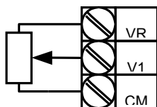
Collegamento del potenziometro ai morsetti VR e CM
