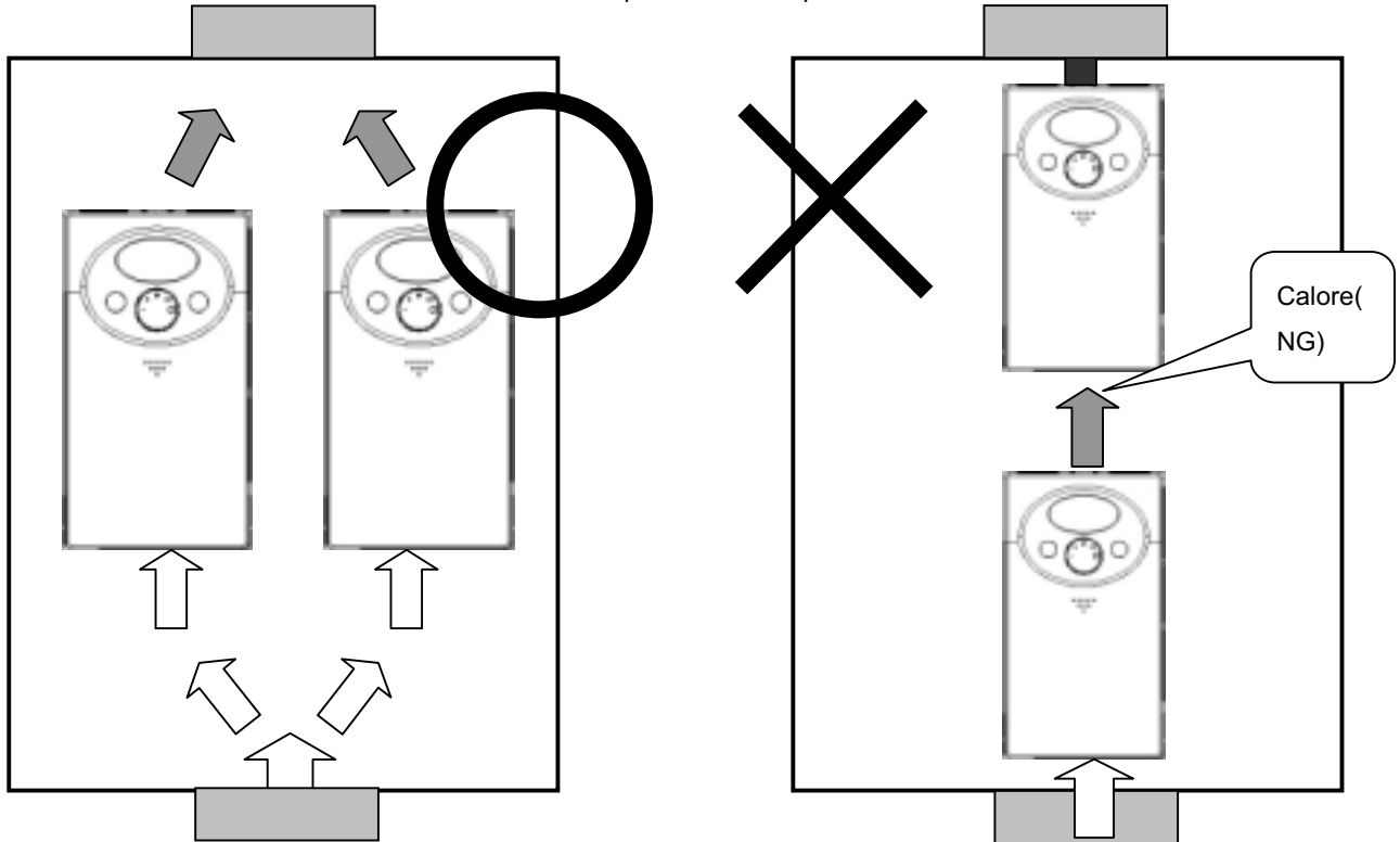
< Installazione di più inverter nel pannello >
